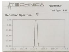
T810 表面式光栅温度传感器由 Technica 公司生产，获 UTC 和 Sylex 公司授权。
